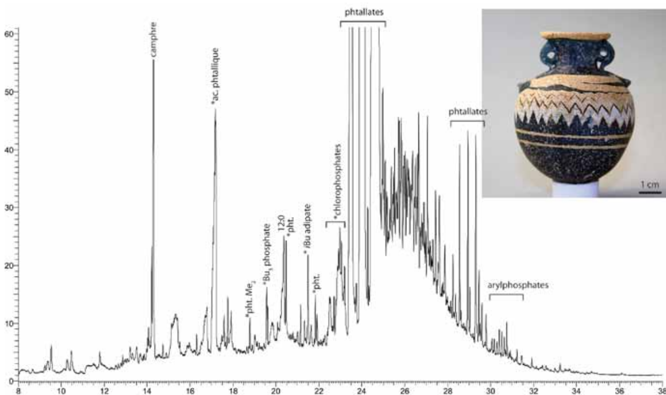
Figure 1 : Chromatogramme de l'extrait lipidique brut du vase 26866.
